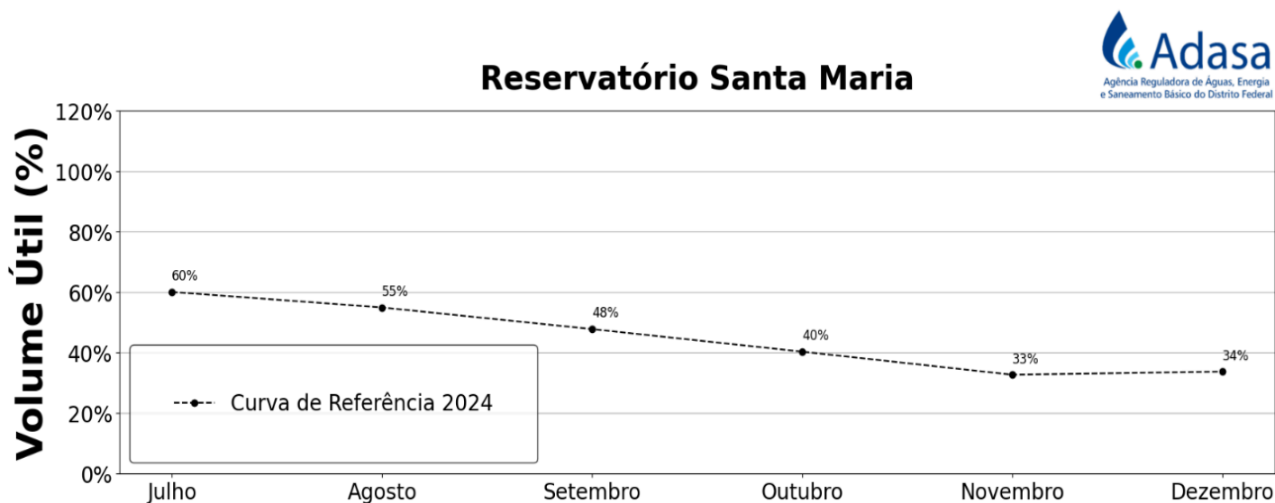
Figura 2 – Curva de referência para o acompanhamento do volume útil do reservatório do Santa Maria no período de julho a dezembro de 2024.
