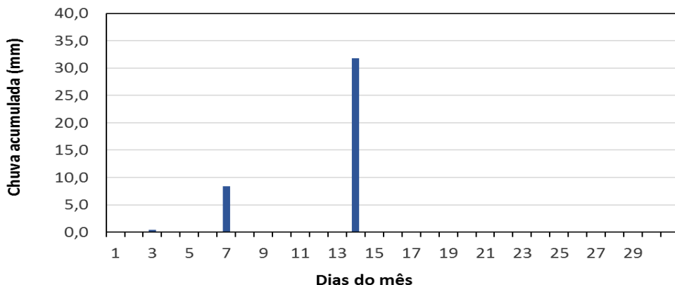
Chuva acumulada no Lago Paranoá - Outubro/2018
