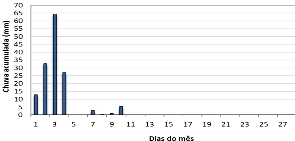
Chuva acumulada no Lago Santa Maria - Fevereiro/2018
