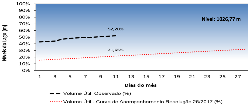
Volume Útil do Lago Descoberto - Fevereiro/2018
