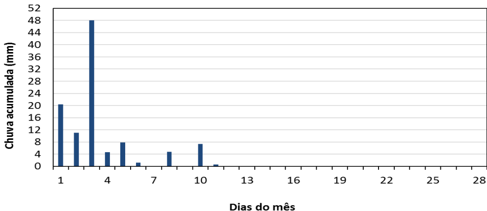
Chuva acumulada no Lago Descoberto - Fevereiro/2018
