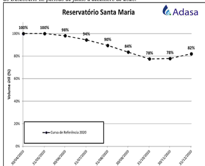
Figura 2 - Curva de referência para o acompanhamento do volume útil do reservatório do Santa Maria no período de junho a dezembro de 2020.
