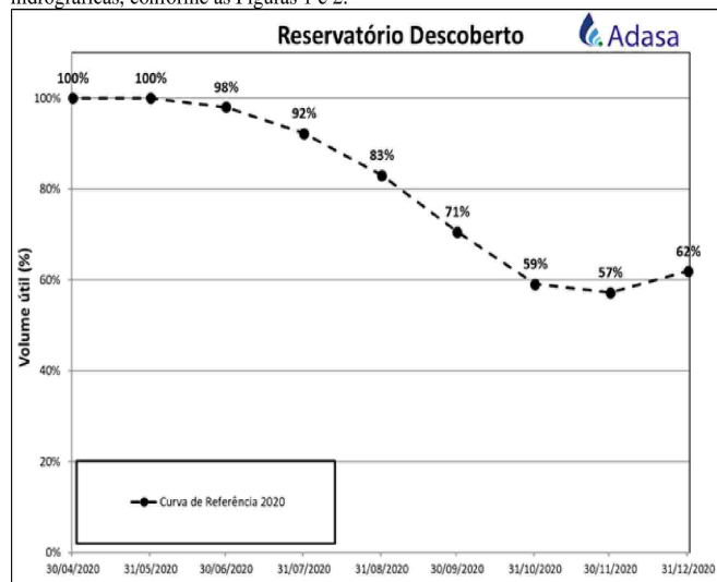
Figura 1 - Curva de referência para o acompanhamento do volume útil do reservatório do Descoberto no período de junho a dezembro de 2020.
