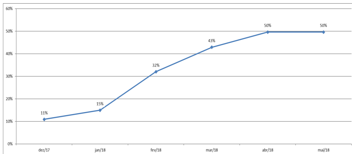
Figura 1 — Curva de acompanhamento do volume útil do reservatório do Descoberto para os meses de janeiro a maio de 2018.
