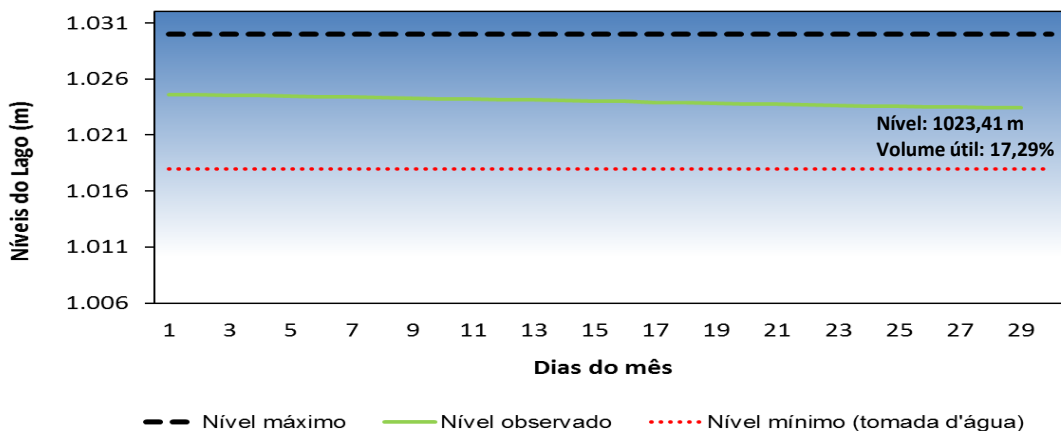
Níveis do Lago Descoberto - Setembro/2017
