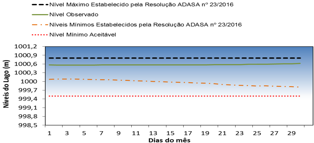
Níveis do Lago Paranoá - Setembro/2017
