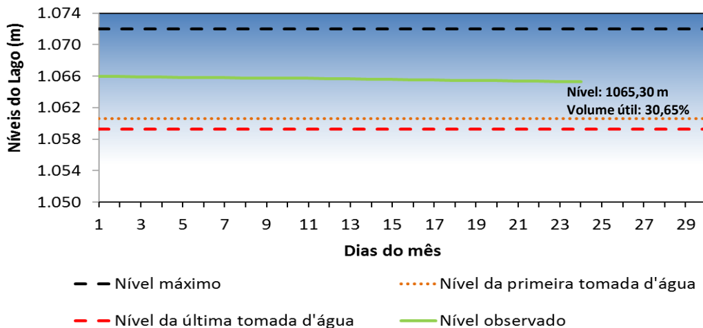
Níveis do Lago Santa Maria - Setembro/2017
