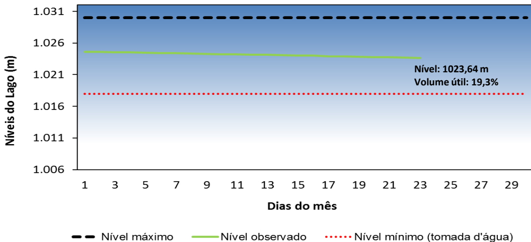
Níveis do Lago Descoberto - Setembro/2017
