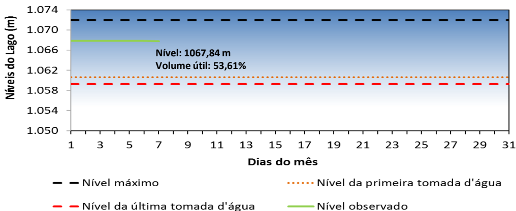
Níveis do Lago Santa Maria - Maio/2017
