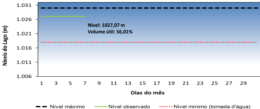
Níveis do Lago Descoberto - Maio/2017
