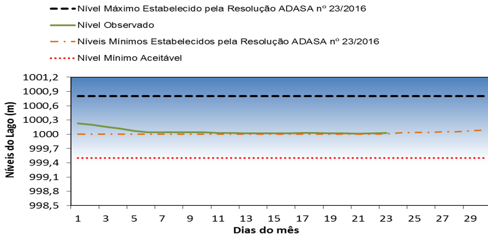
Níveis do Lago Paranoá - Abril/2017
