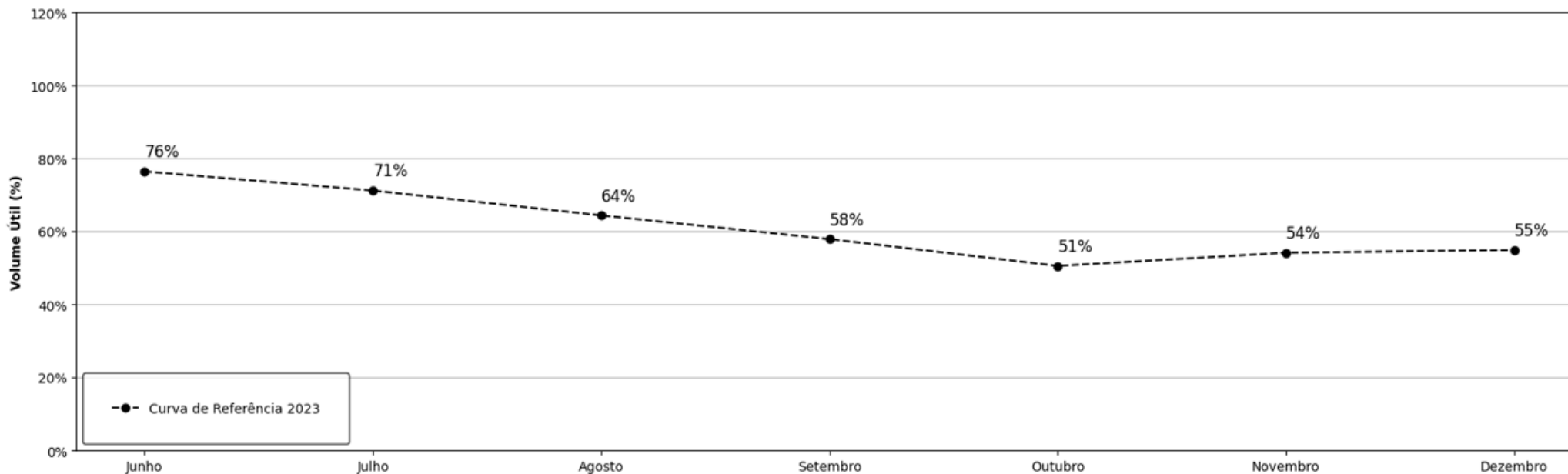
Figura 2 – Curva de referência para o acompanhamento do volume útil do reservatório do Santa Maria no período de julho a dezembro de 2023.
