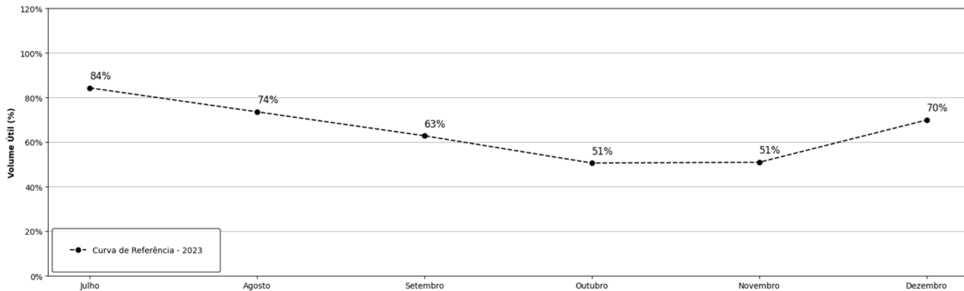
Figura 1 – Curva de referência para o acompanhamento do volume útil do reservatório do Descoberto no período de julho a dezembro de 2023.
