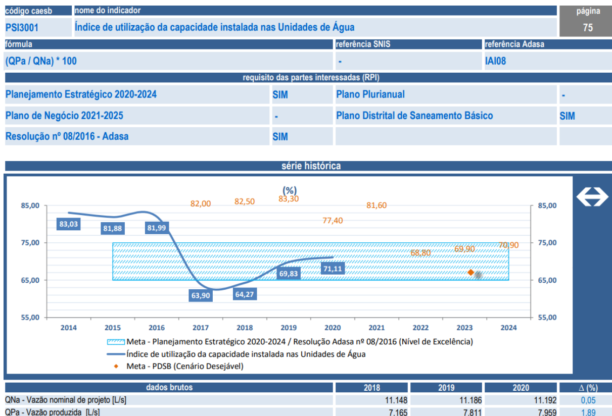
Figura 27: Capacidade instalada nas Unidades de Água. (Fonte: Relatório de Indicadores da Caesb/2020).
