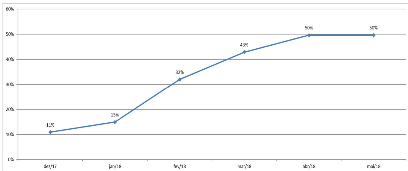
Figura 1 - Curva de acompanhamento de metas para o volume útil do reservatório do Descoberto nos meses de janeiro a maio de 2018.
