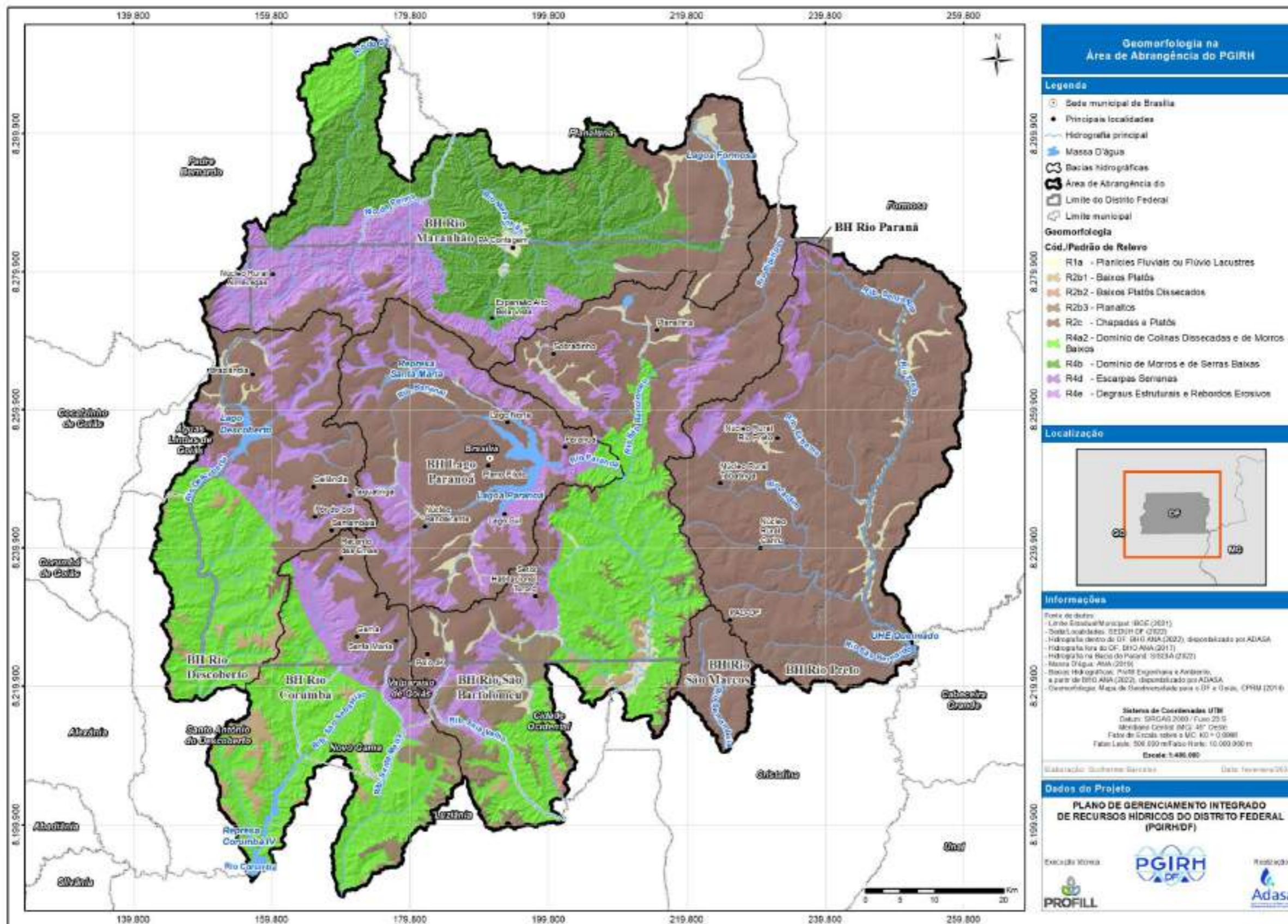
Figura 3.11 - Geomorfologia na área de abrangência do PGIRH/DF.
