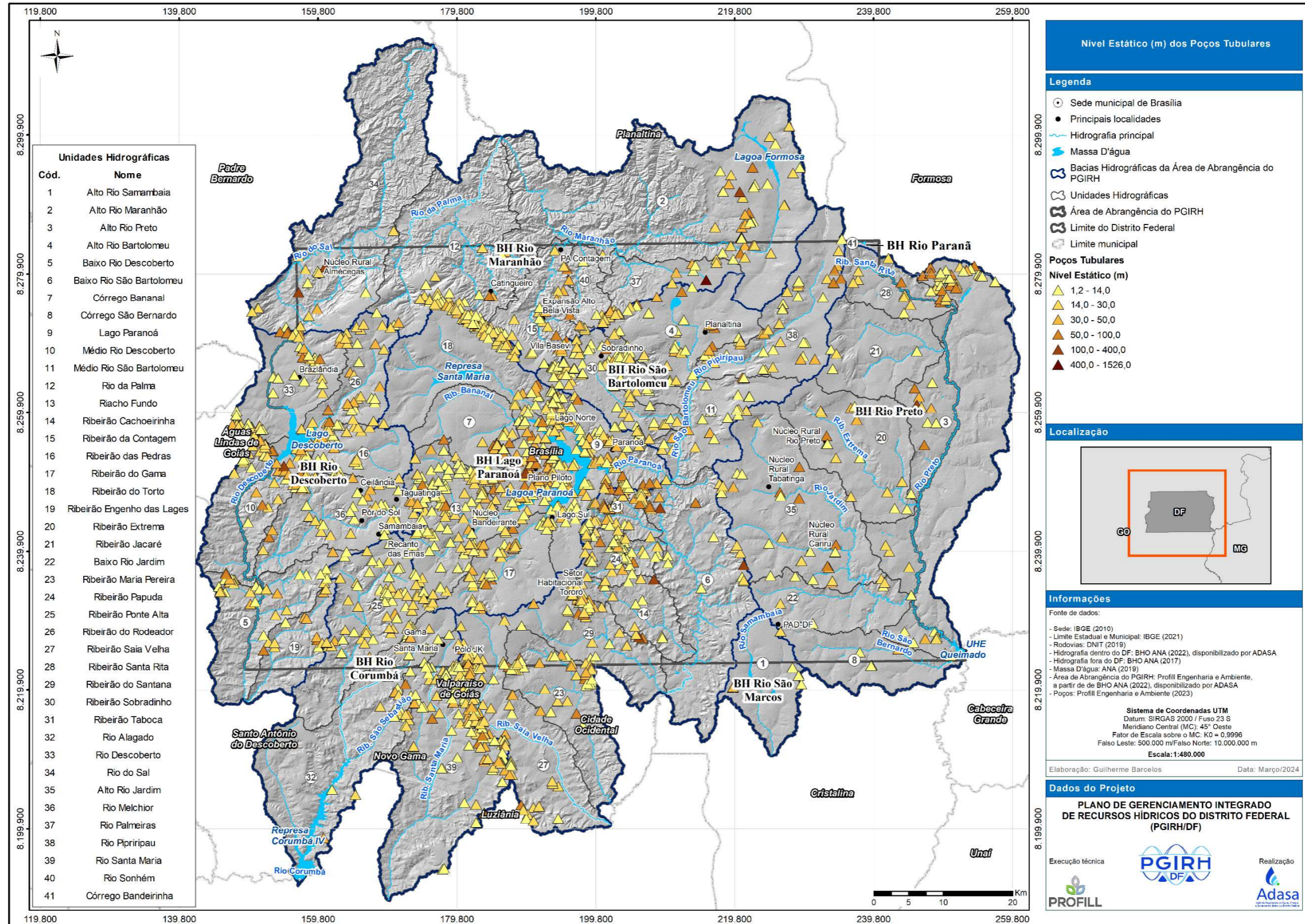
Figura 12.8 - Nível estático (m) dos poços tubulares.
