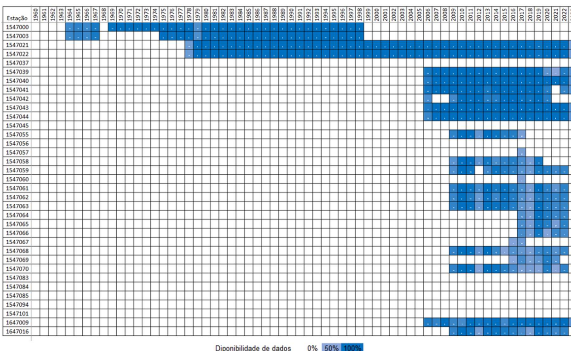
Figura 11.39 - Disponibilidade de dados de precipitação na bacia hidrográfica do rio Preto.
