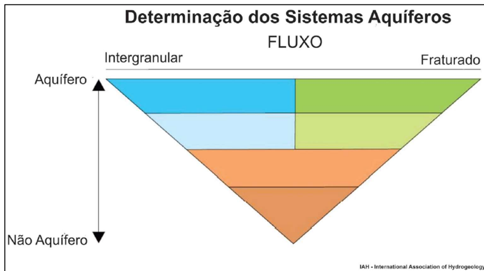
Figura 12.3 - Classificação da produtividade dos aquíferos. Fonte: SGB (2014).
