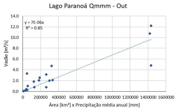
Figura 11.17 - Regionalização vazões de referência Rio Paranoá - B. Fonte: Elaboração própria, 2024.
