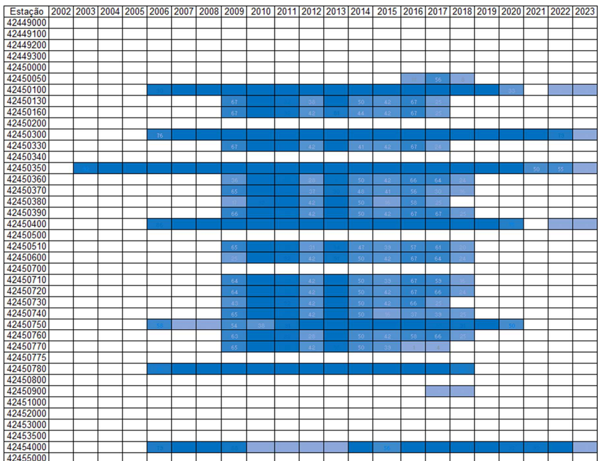
Figura 11.41 - Disponibilidade de dados de vazão na bacia hidrográfica do rio Preto.
