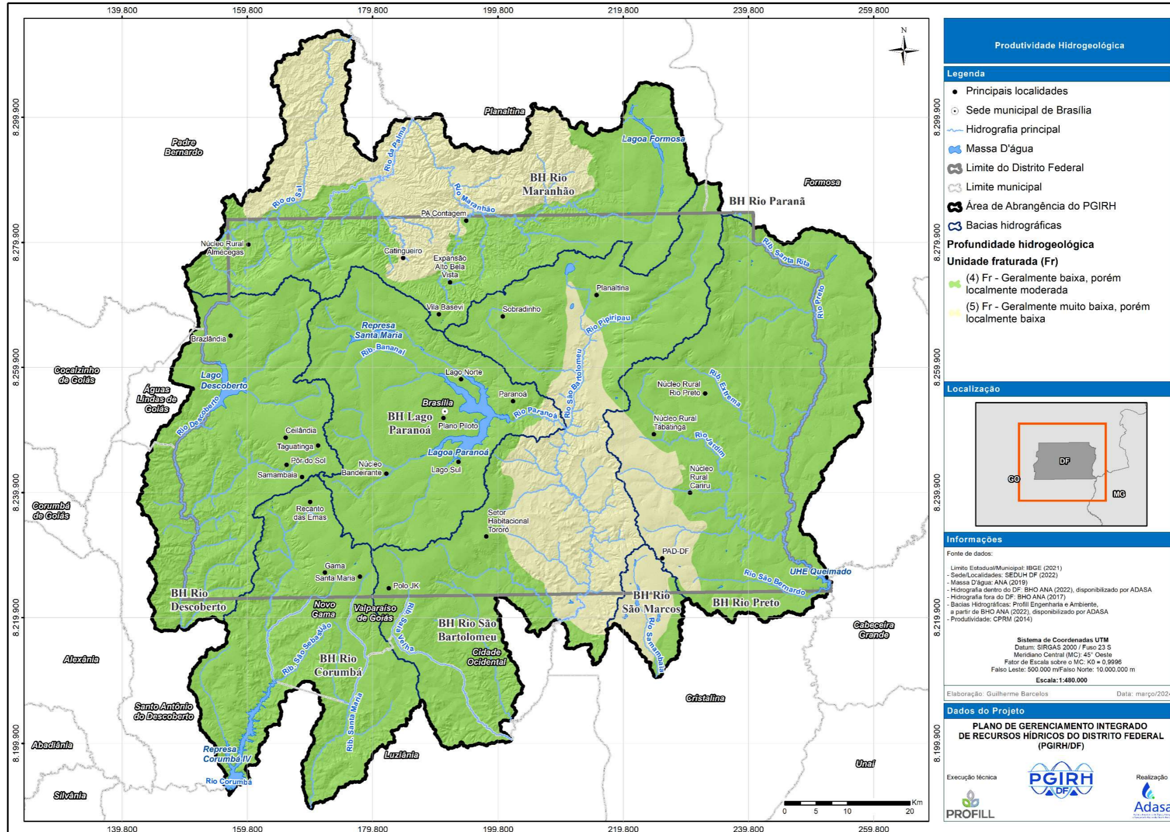
Figura 12.4 - Classificações de Produtividade. Fonte: Diniz et al. (2014).
