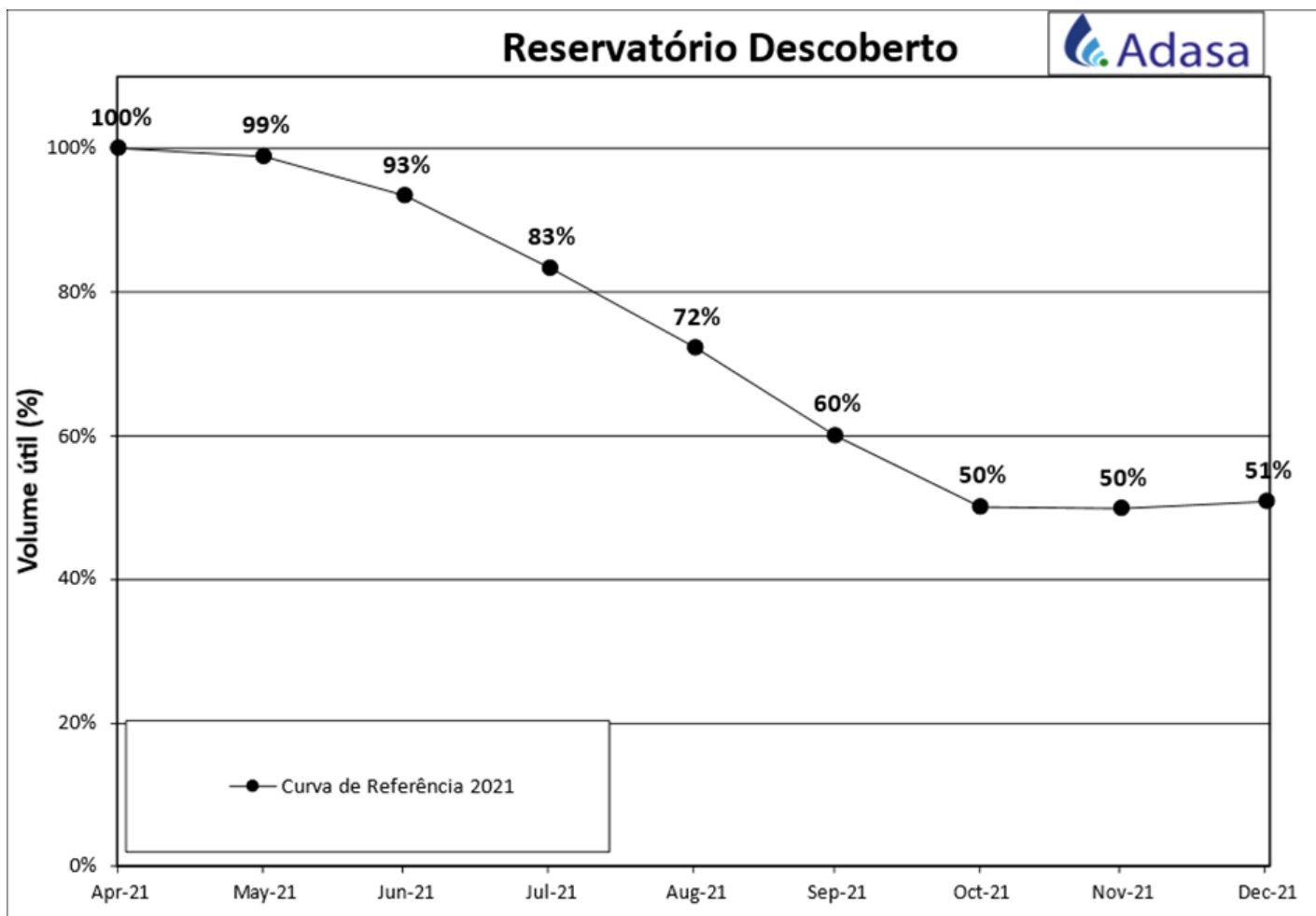
Figura 1 – Curva de referência para o acompanhamento do volume útil do reservatório do Descoberto no período de junho a dezembro de 2021.
