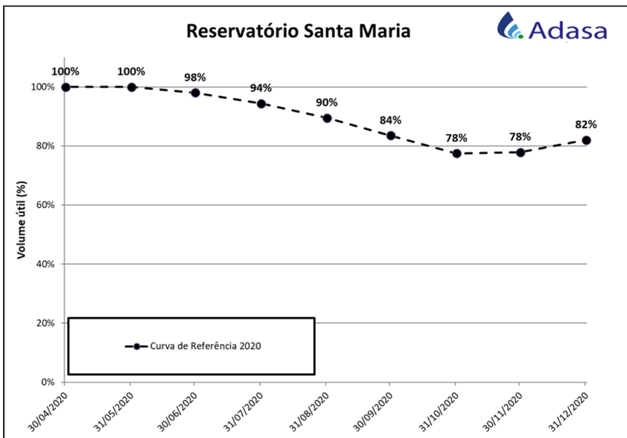
Figura 2 - Curva de referência para o acompanhamento do volume útil do reservatório do Santa Maria no período de junho a dezembro de 2020.
