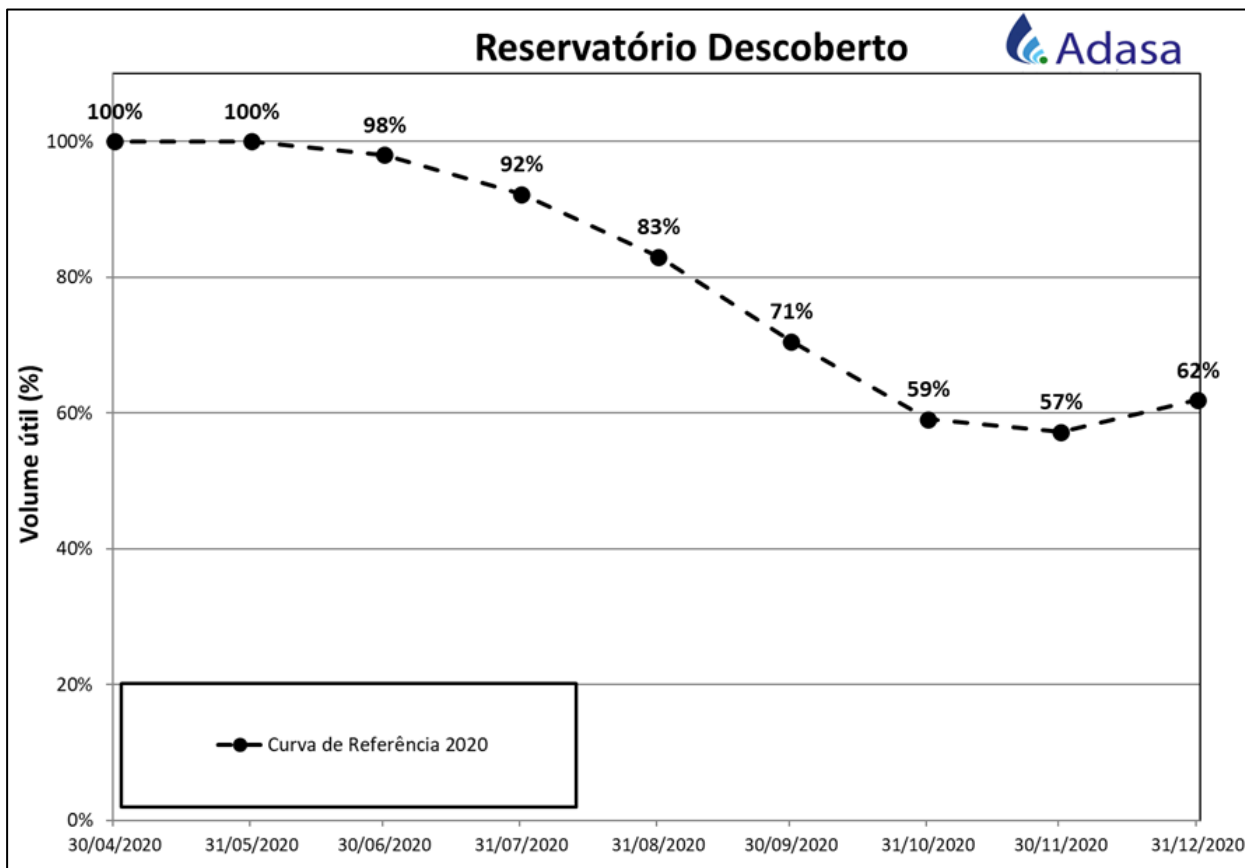
Figura 1 - Curva de referência para o acompanhamento do volume útil do reservatório do Descoberto no período de junho a dezembro de 2020.
