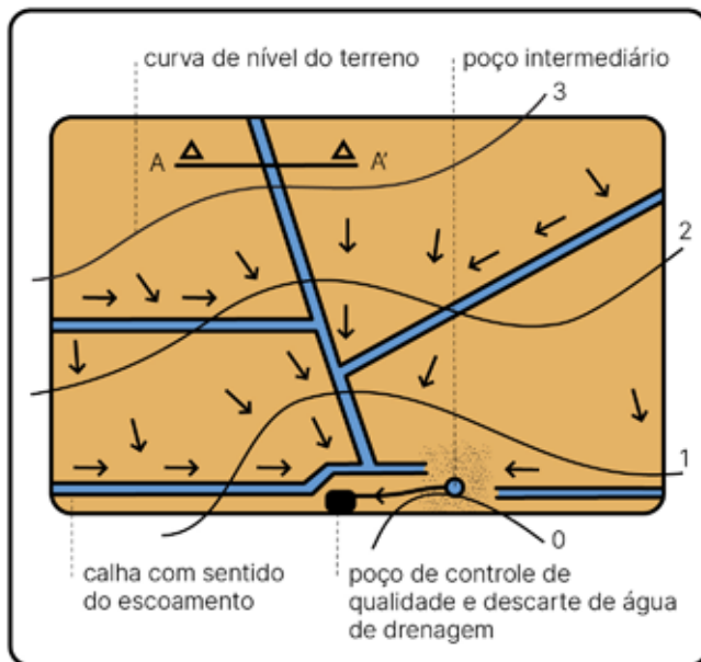
Esquema 14 Alternativa 3 - Terreno hipotético com caminho de água preferencial no centro. Fonte: Rosa (2019)
