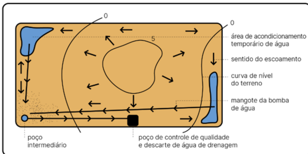
Esquema 15 Alternativa 4 - Terreno hipotético com divergência dos fluxos de água. Fonte: Rosa (2019)
