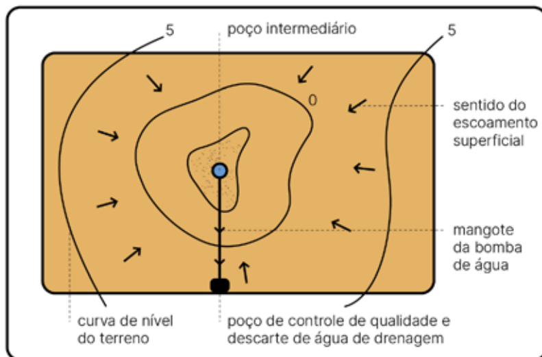
Esquema 16 Alternativa 4 - Terreno hipotético com convergência dos fluxos de água. Fonte: Rosa (2019)
