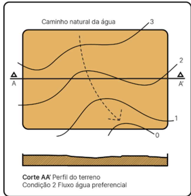
Esquema 5 Condição topográfica 2, terreno com caminho natural da água pré-existente. Fonte: Rosa (2013)
