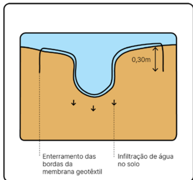
Detalhe 13 Corte AA' da calha provisória do Esquema 14. Fonte: Rosa (2019)
