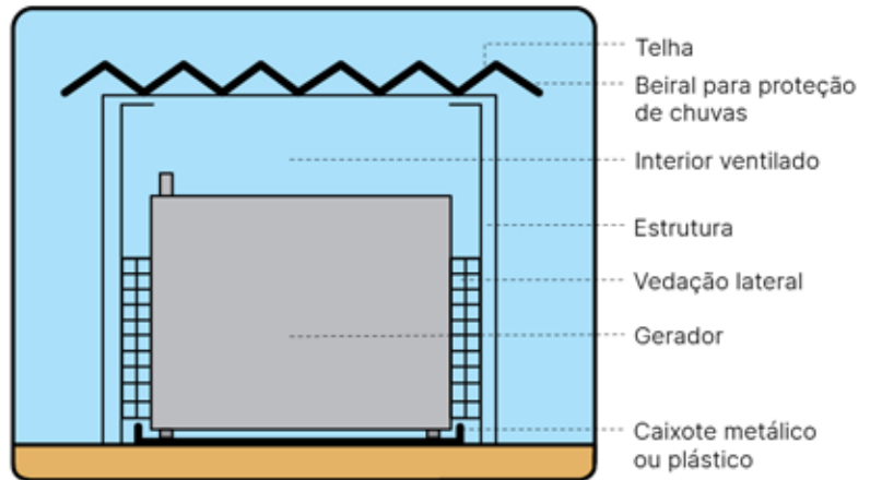
Corte Gerador protegido contra intempéries e contaminação do solo e água
