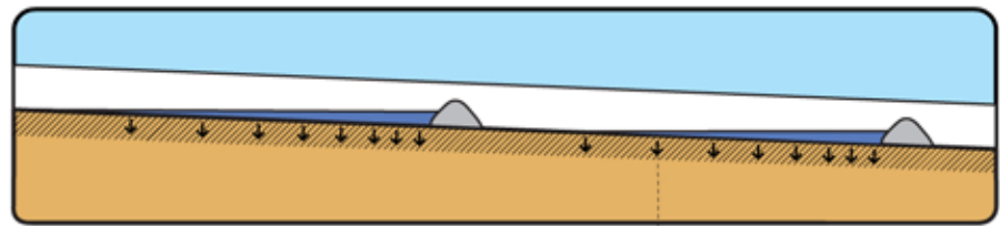
Corte AA' Perfil longitudinal da calha demonstrando barreiras de sedimentos sequenciais Infiltração de água no solo
