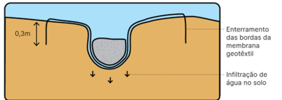
Corte BB' Perfil da calha com barreira de sedimentos
