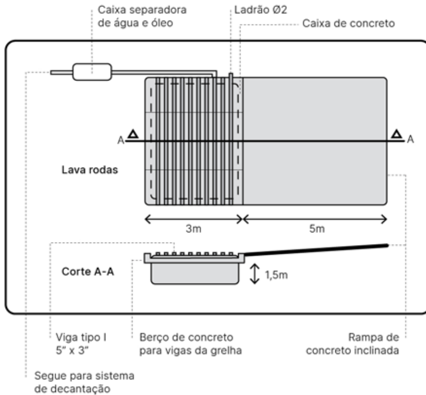
Figura 29 Projeto lava rodas. Fonte: Abreu e Souza (2012)
