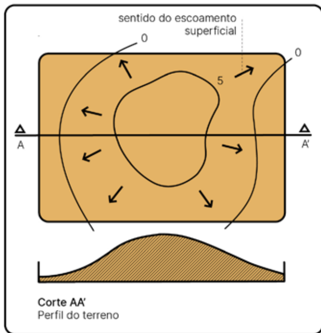
Esquema 10 Identificação das áreas de contribuição em terrenos com divergência de águas. Fonte: Rosa (2019)
