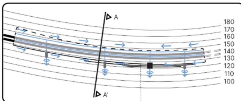
Planta baixa Projeto de drenagem do canteiro de obras de serviços
