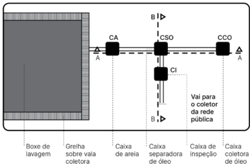
Figura 30 Croqui do sistema Separador Água-Óleo adotado (Caixa de inspeção interligada com sistema de drenagem). Fonte: CAESB (2020)
