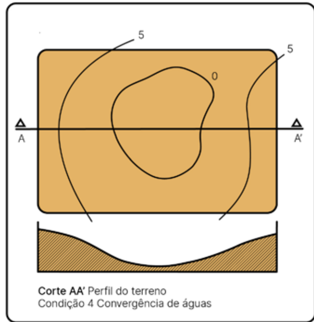
Esquema 7 Condição topográfica 4, terreno com convergência de águas. Fonte: Rosa (2013)
