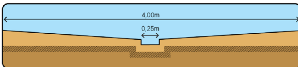
Corte AA' Transversal Caimento da superfície sentido centro longitudinal
