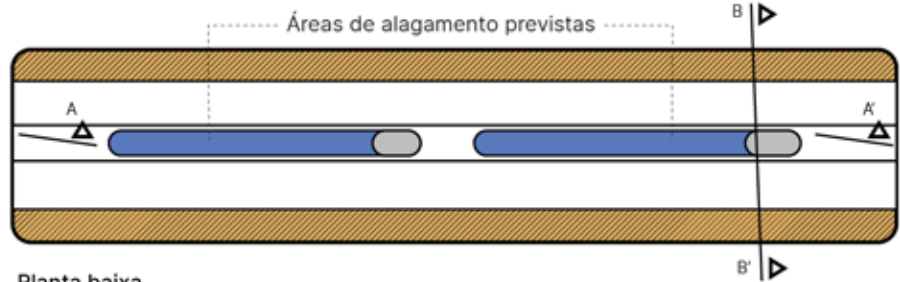
Planta baixa Vista superior da calha barreiras de sedimentos
