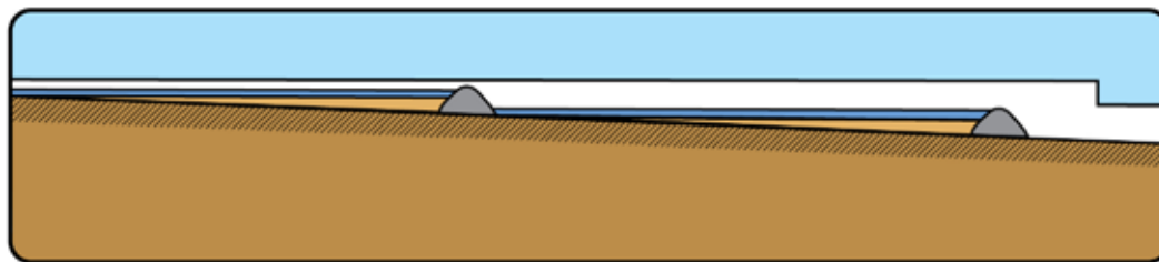
Corte BB' Longitudinal Barreiras de sedimentos com sacarias de rafia ou membrana geotêxtil preenchidas com agregados dispostas no interior da calha do sistema lava rodas auxiliam no tratamento da água de lavagem.
