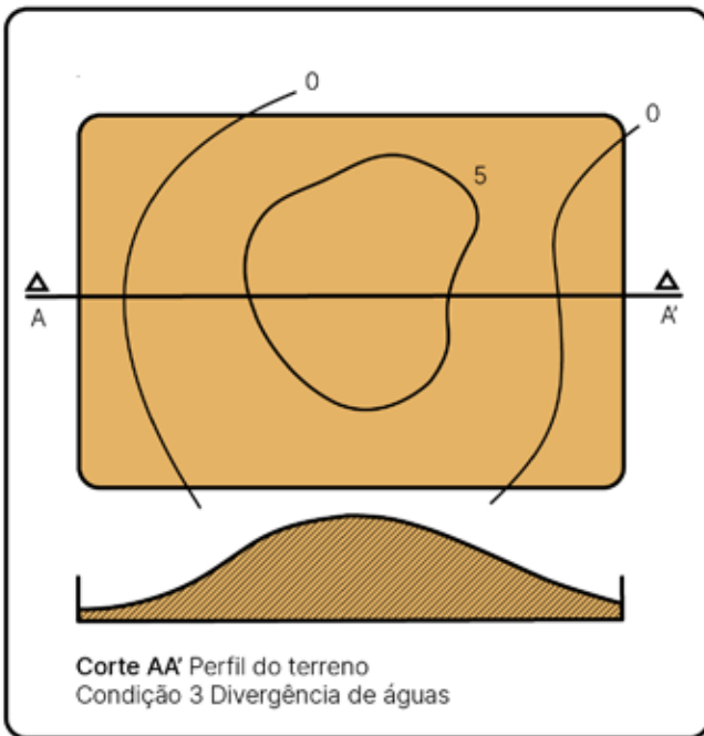
Esquema 6 Condição topográfica 3, terreno com divergência de águas. Fonte: Rosa (2013)
