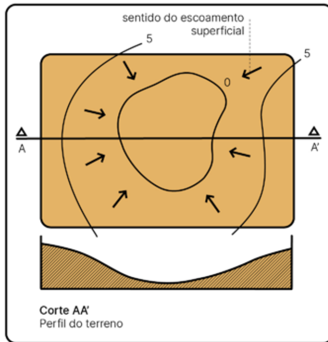
Esquema 11 Identificação das áreas de contribuição em terrenos com convergência de águas. Fonte: Rosa (2019)
